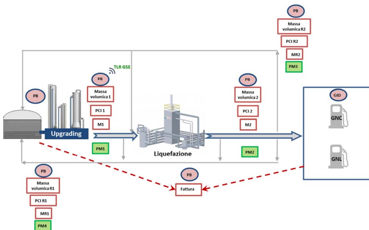
Figura 13 – Schema dei punti di misura e delle grandezze rilevanti ai fini del calcolo della quantità ammissa all'incentivo nel caso di immissione in consumo del biometano in forma liquida (BML) tramite connessione diretta all'impianto di liquefazione e a quello di distribuzione, senza ritiro del biometano da parte del GSE.
