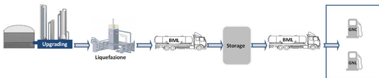
Figura 12- Configurazione NON ammessa secondo quanto riportato al vincolo 3 relativo alla configurazione 5
