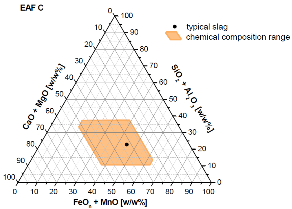
Figura 1 – Diagramma ternario della scoria EAF-C.
